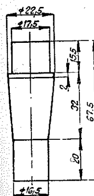
Súčiastka A zo zostavy 13a
