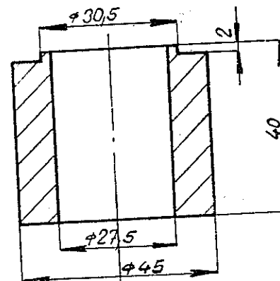
Súčiastka B zo zostavy 13a
