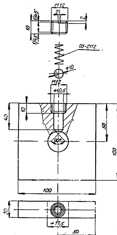
Súčiastka C zo zostavy 13b
