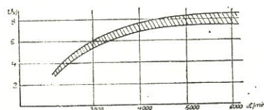
Obr. 38. Závislosť napätia od obrátok alternátora. Zataženie žiarovkami 5 + 25 W.
